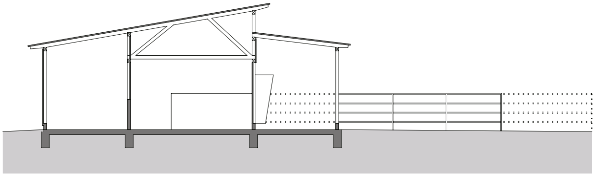
SCHNITT
